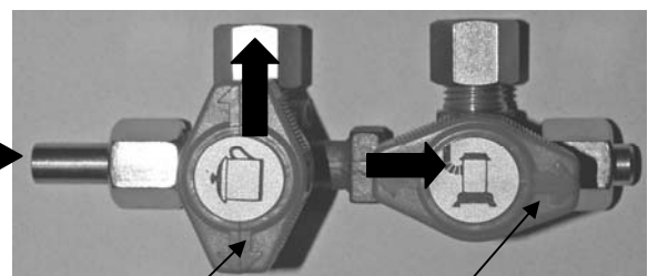
Hahn offen
